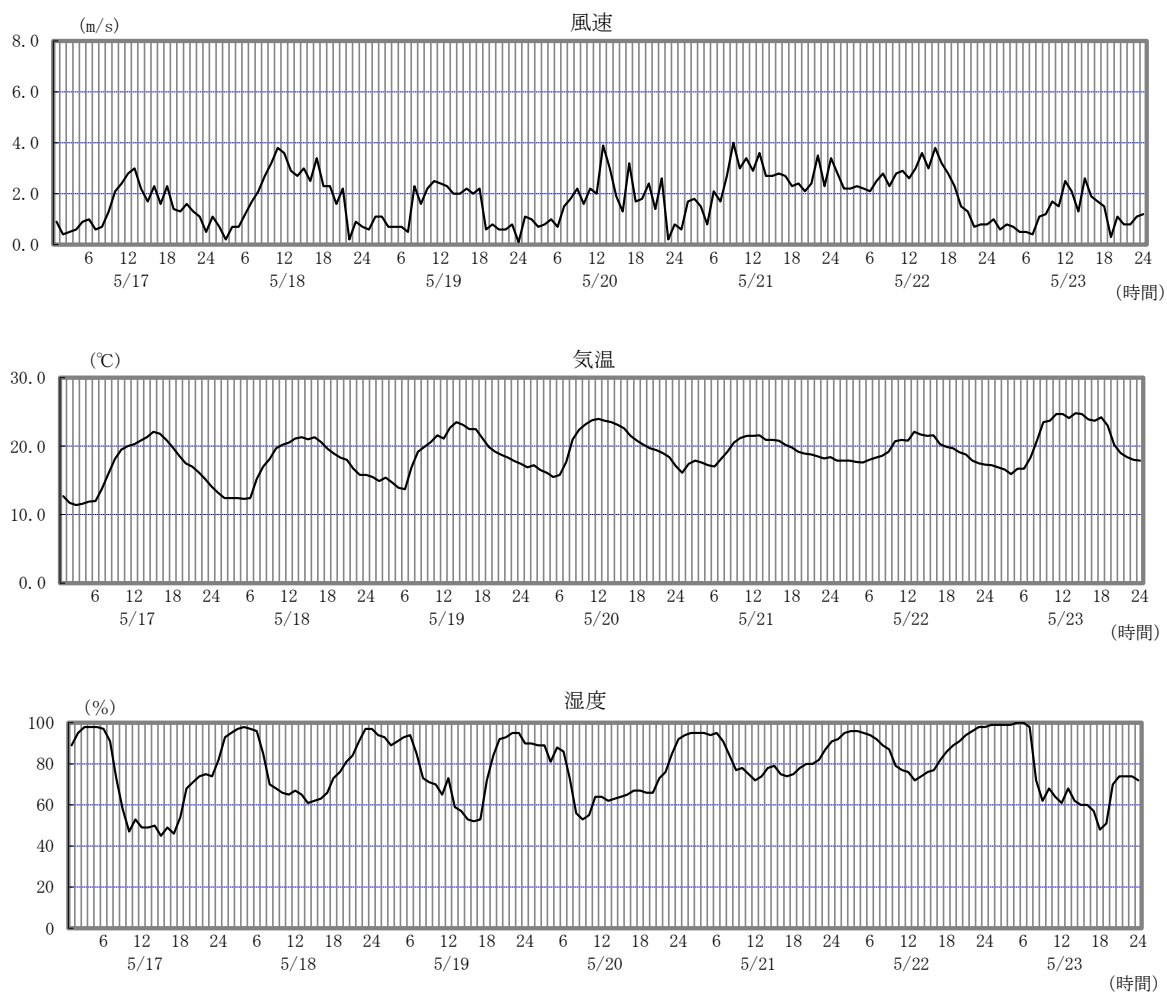
図 3-2-2 屋形石公民館 気象調査結果
