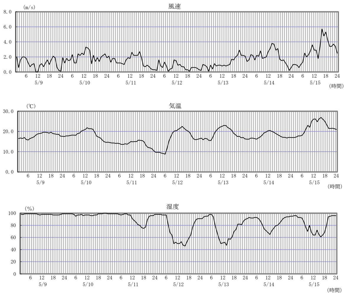
図 3-2-3 打上小学校 気象調査結果
