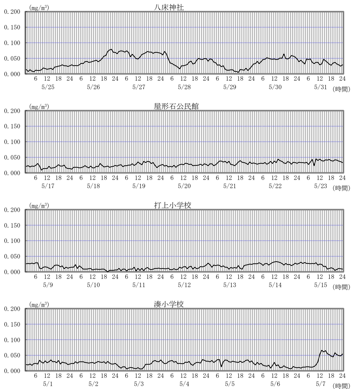
図 3-3-5 浮遊粒子状物質測定結果
