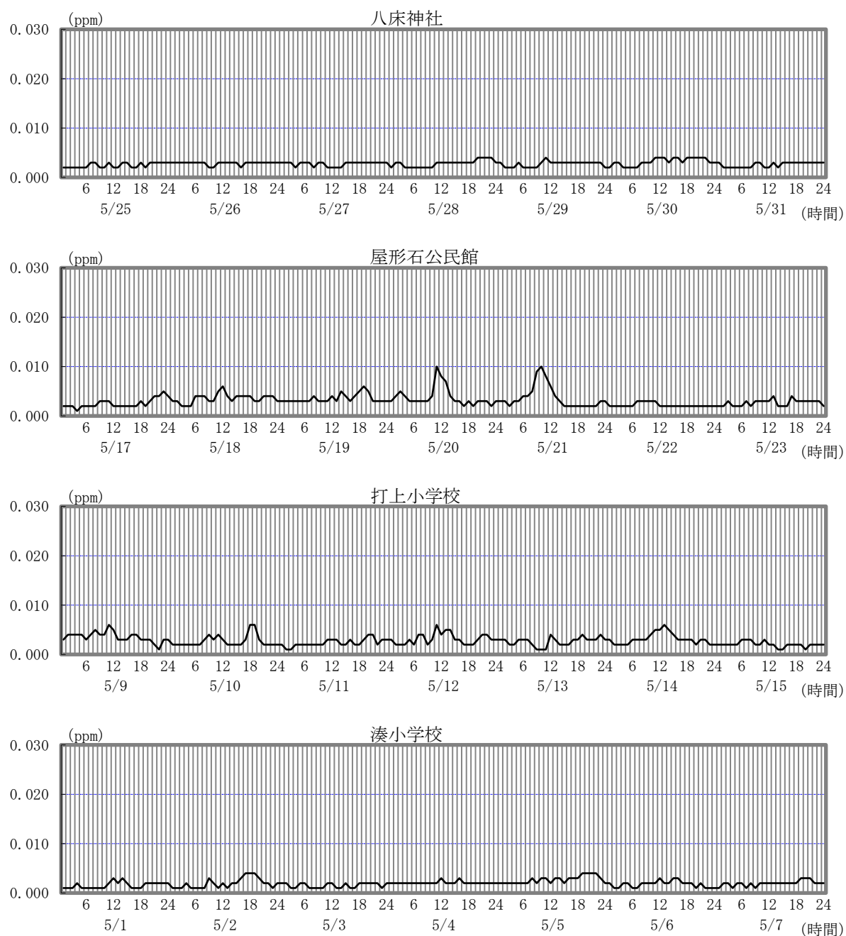
図 3-3-3 二酸化窒素測定結果
