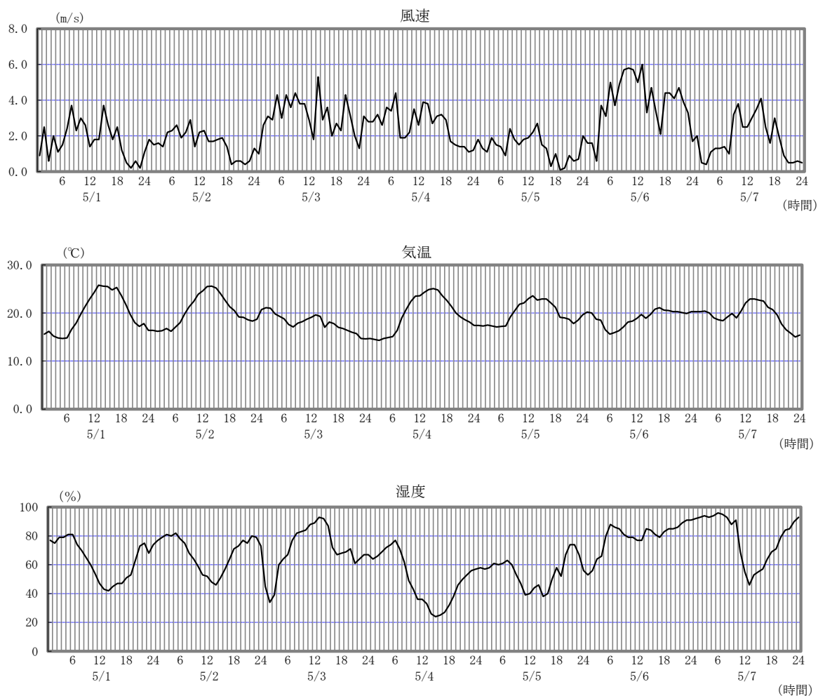
図 3-2-4 湊小学校 気象調査結果
