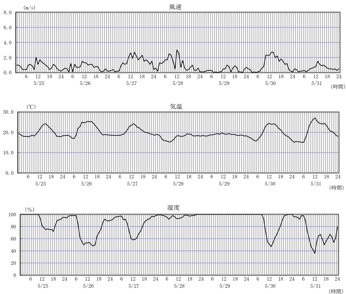
図 3-2-1 八床神社 気象調査結果
