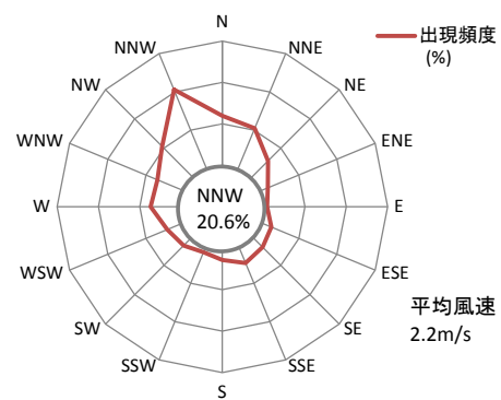
図 3-2-6 気象観測集計結果 (2/2)
