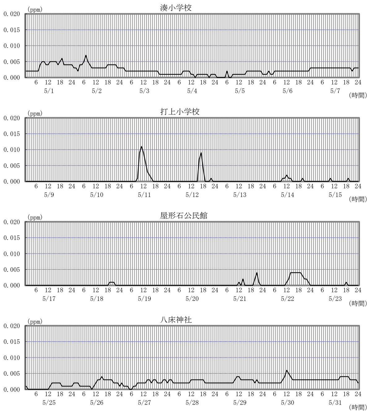
図 3-3-1 二酸化硫黄測定結果
