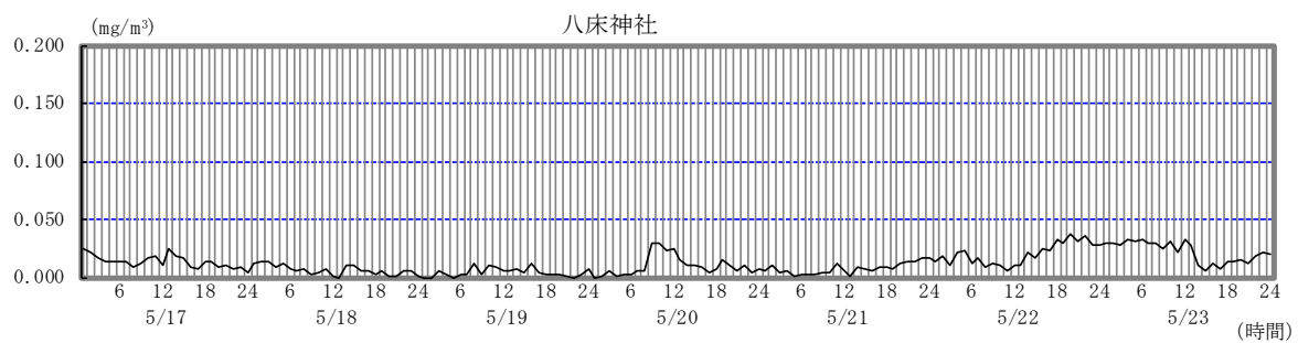
図 3-3-5 浮遊粒子状物質測定結果
