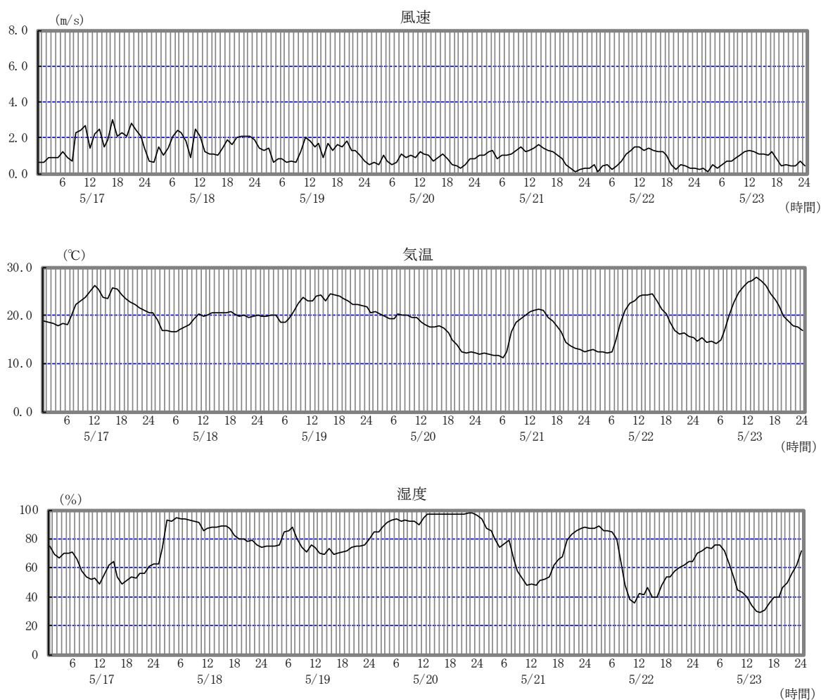
図 3-2-4 八床神社 気象調査結果
