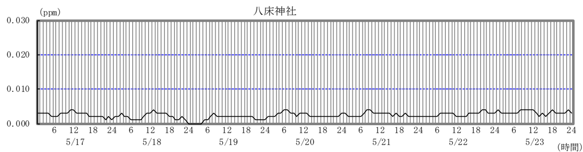
図 3-3-3 二酸化窒素測定結果
